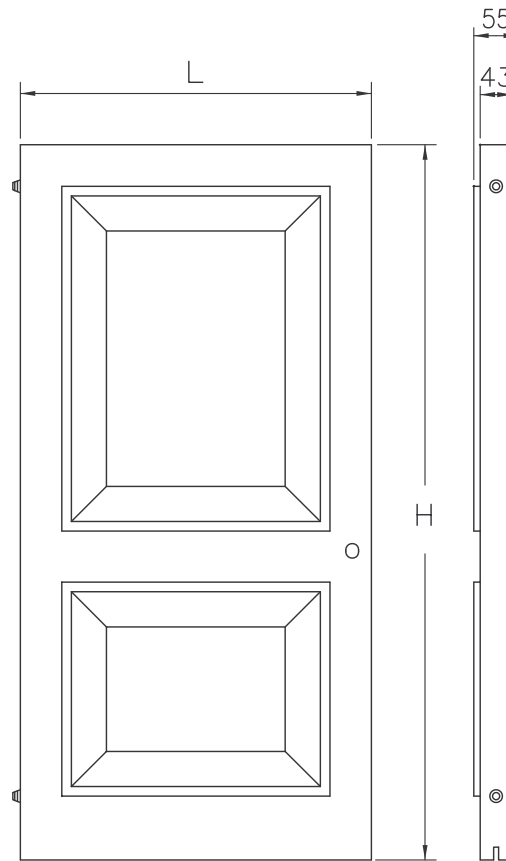
DIMENSIONI PANNELLO-DIMENSIONS DES PORTES-MEDIDAS DE LAS HOJAS-TÜRMASS-DOOR DIMENSIONS
